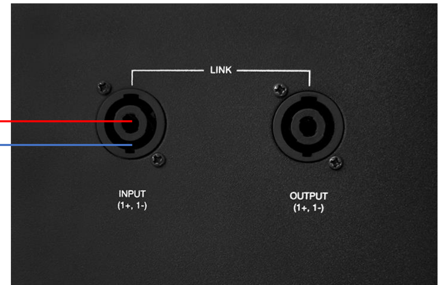
SOUND8 esempio di collegamenti a 8 Ω
