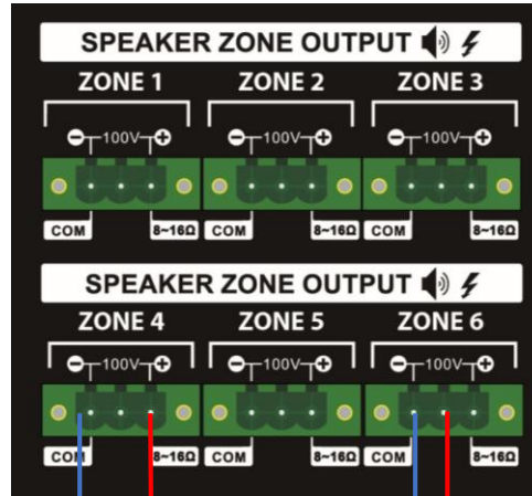
FLORA16T esempio di collegamenti a 100V
