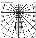
mod.M3 Spot 36°
