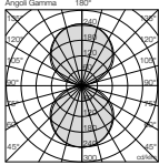
mod.BS Biemissione 120°
