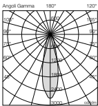
mod.M3 Spot 36°
