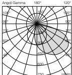
mod.AR Asimmetrico 45°
