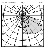
mod.AR Asimmetrico 45°
