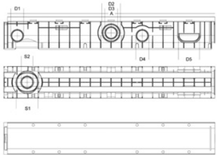
Caniveau PP bordure en acier
