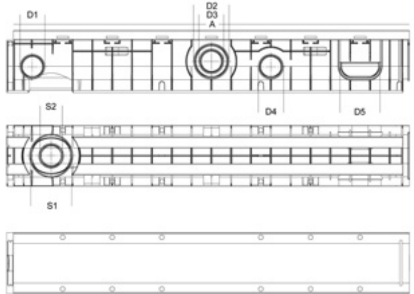
Caniveau PP bordure en acier
