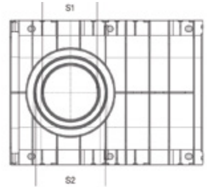
Canal de PP con bordes de acero
