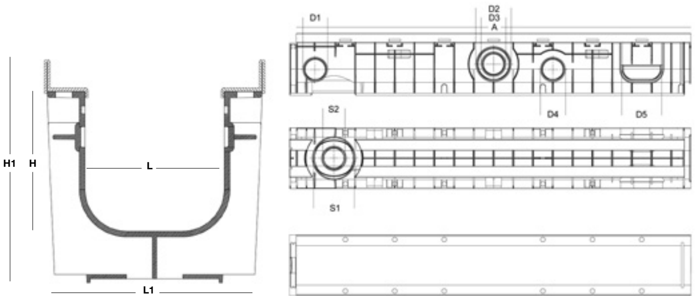
Canale PP con bordi in acciaio
